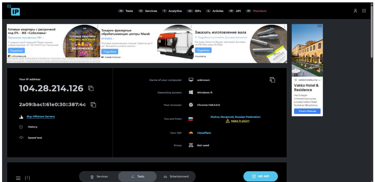
Скриншот: test1_main_page.png
