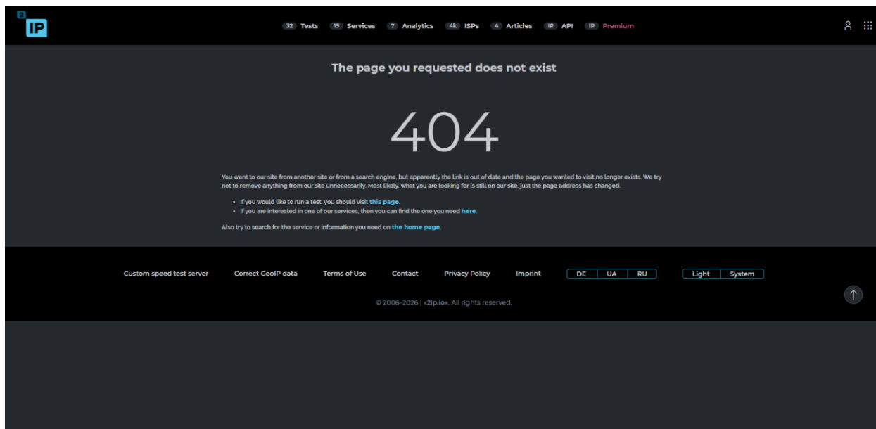
Скриншот: test3_404.png
