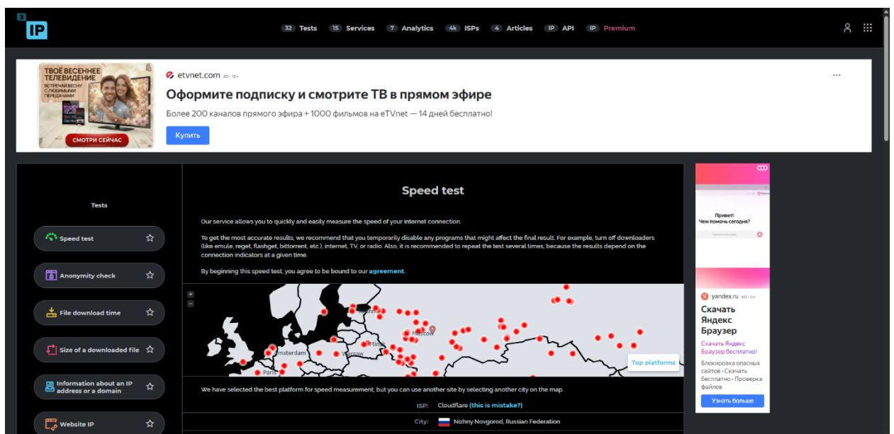
Скриншот: test2_speed_page.png
