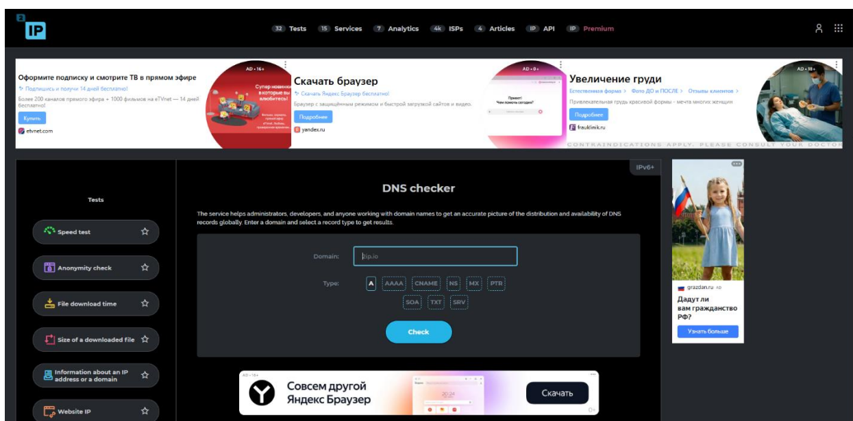
Скриншот: test4_dns_before.png
