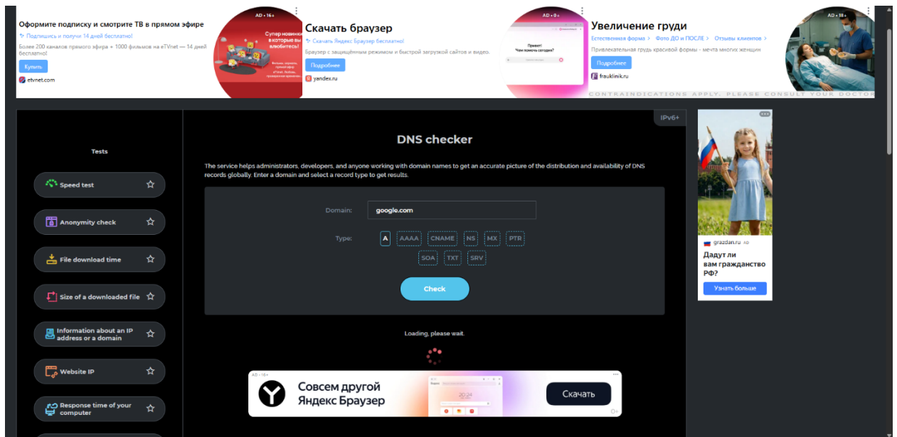
Скриншот: test4_dns_success.png
